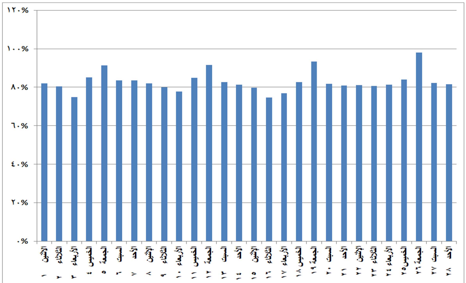
شكل (٢٨) نسب الفائض للحمل الاقصى المسجل يوميا خلال شهر فبراير ٢٠٢١
