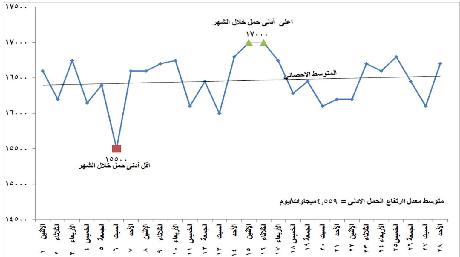
شكل (٢) تطور الحمل الادنى اليومي خلال شهر فبراير ٢٠٢١
