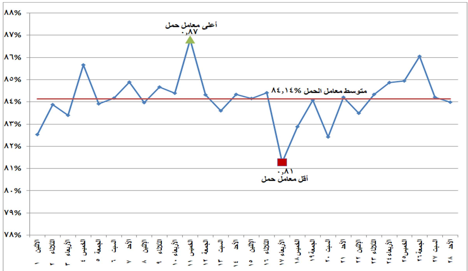
شكل (١٢) إجمالي معامل الحمل لوحدات الانتاج خلال شهر فبراير ٢٠٢١
