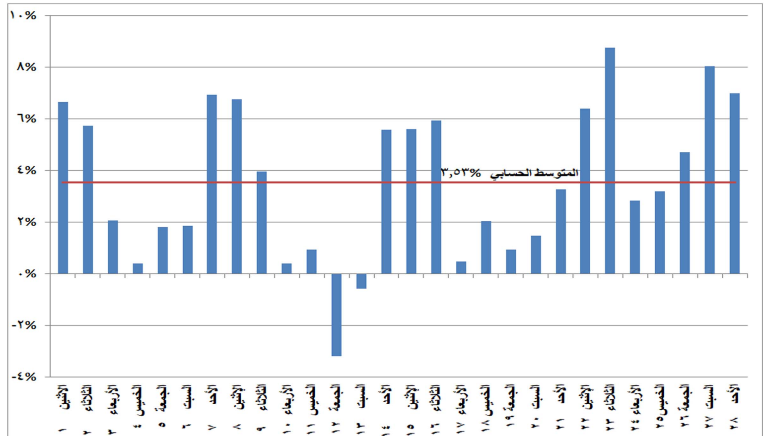
شكل (١٧) الطاقة الكهربائية المنتجة من الغاز الطبيعي خلال شهر فبراير ٢٠٢١
