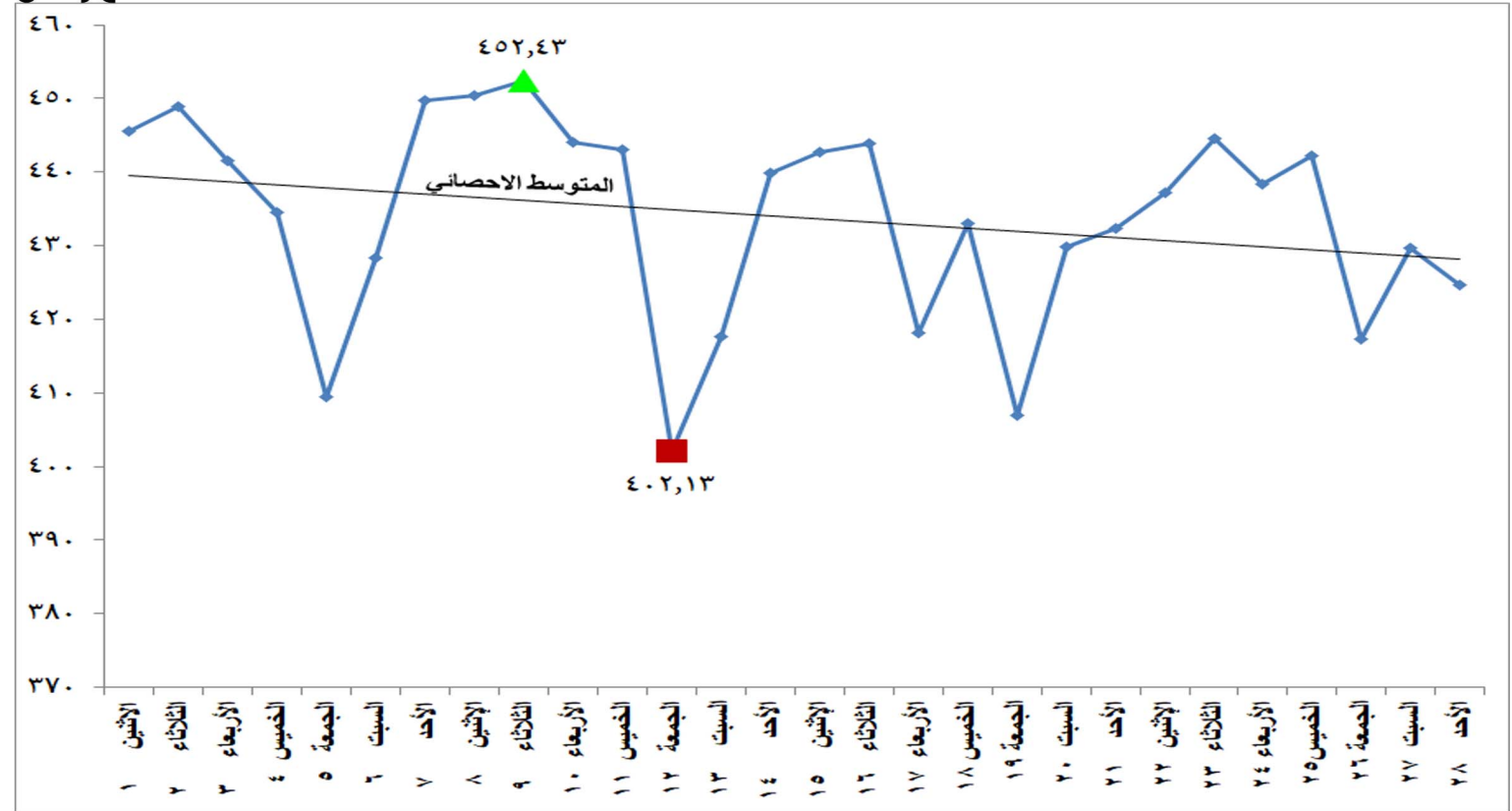
شكل (١٧) الطاقة الكهربائية المنتجة من الغاز الطبيعي خلال شهر فبراير ٢٠٢١
