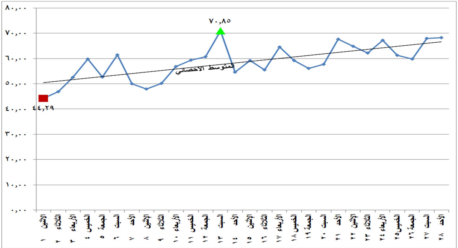
شكل (٢١) الطاقة الكهربائية المنتجة من المصادر غير الحرارية خلال شهر فبراير ٢٠٢١
