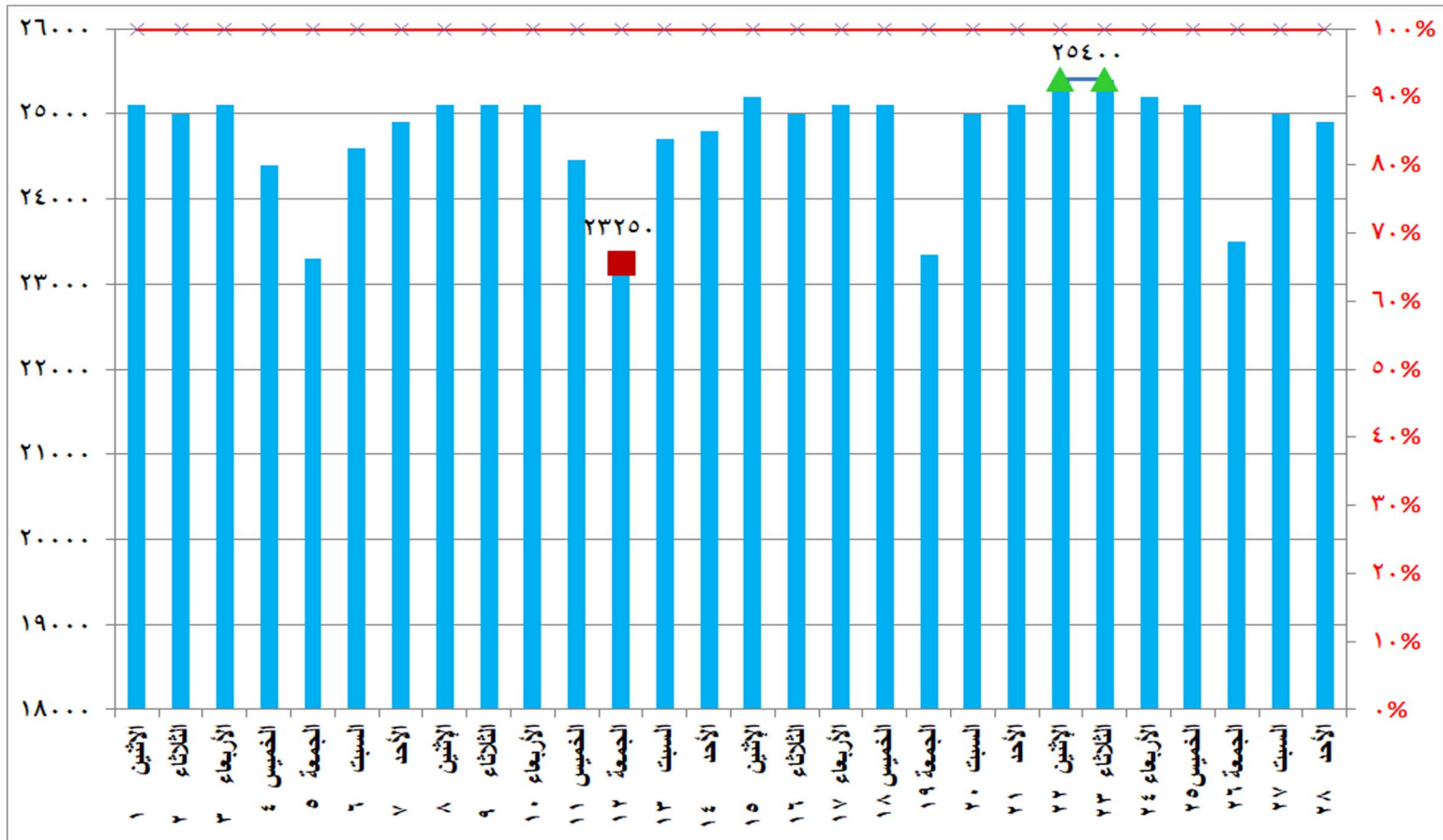
شكل (٥) قدرات الانتاج المتاحة ونسبتها للحمل الأقصى خلال شهر فبراير ٢٠٢١
