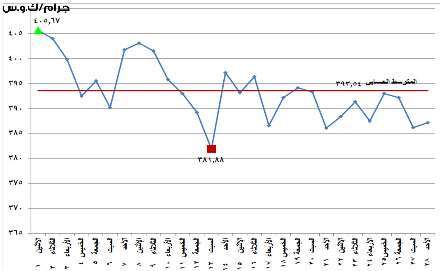
شكل (١٤) معامل انبعاثات غاز ثاني اكسيد الكربون المكافئ على مدى شهر فبراير ٢٠٢١
