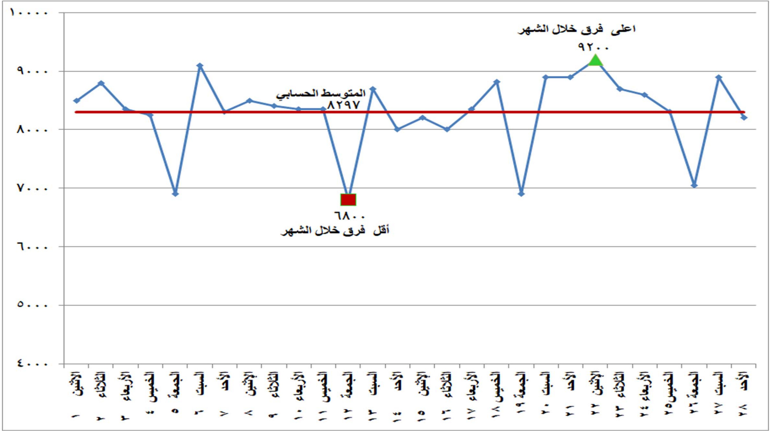
شكل (٣) الفرق بين أقصى وأدنى حمل خلال شهر فبراير ٢٠٢١
