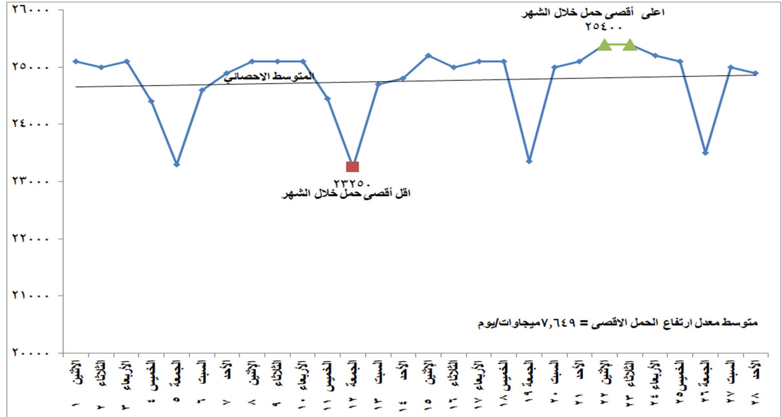
شكل (١) تطور الحمل الاقصى اليومي خلال شهر فبراير ٢٠٢١
