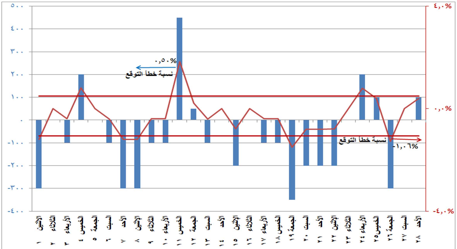
شكل (١٠) الفرق بين الحمل الأقصى المتوقع والمسجل فعليا ونسبة الفرق إلى الحمل المسجل فعليا خلال شهر فبراير ٢٠١٩
