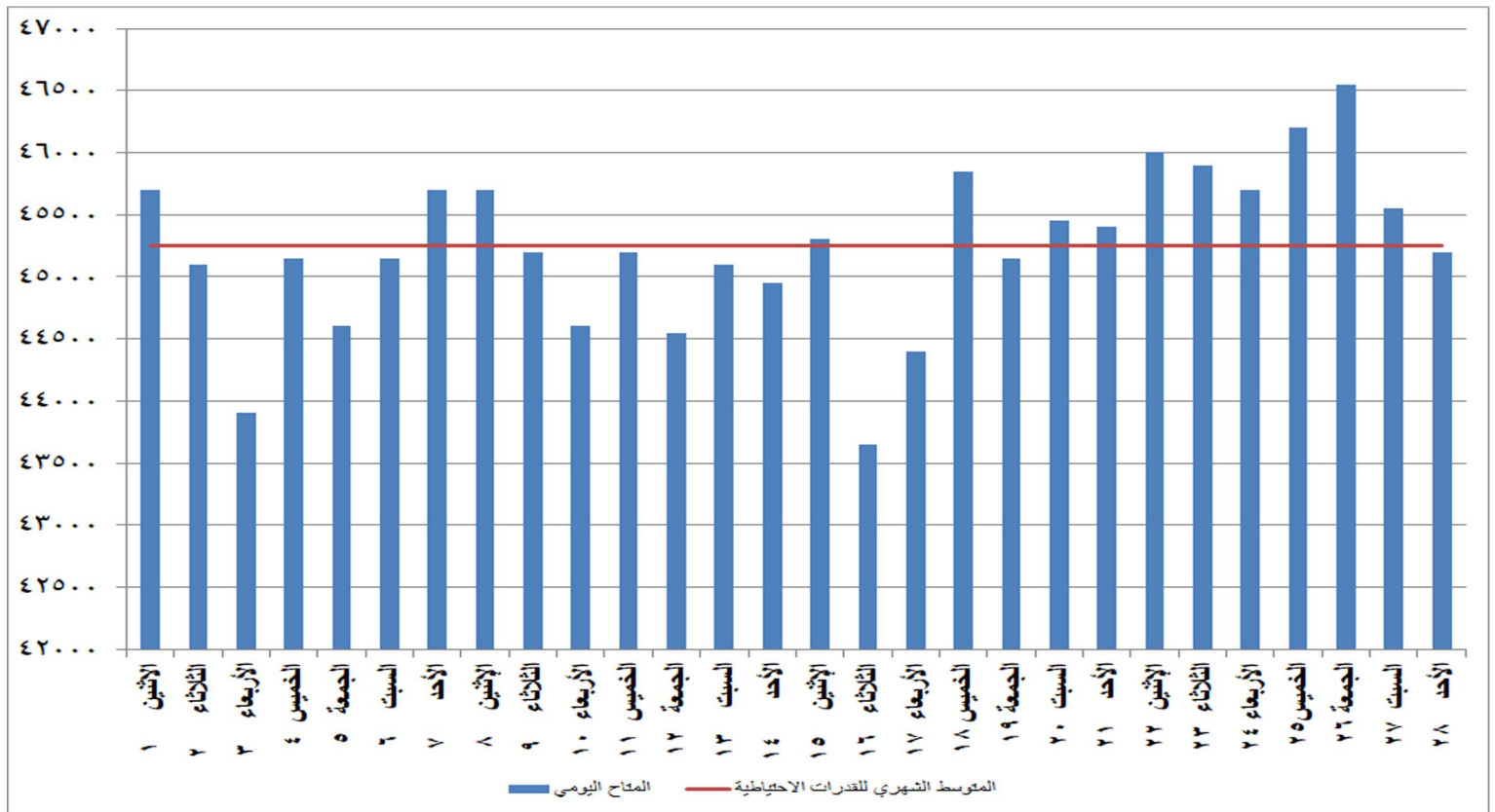
شكل (٢٧) القدرات المتاحة يوميا والمتوسط الشهري للقدرة الاحتياطية خلال شهر فبراير ٢٠٢١
